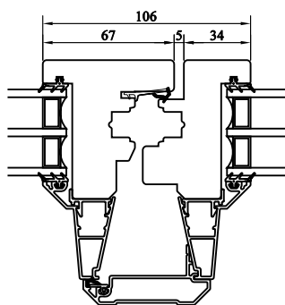
Horizontalsnitt pardörr
