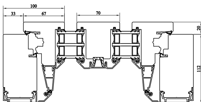
Horizontalsnitt
