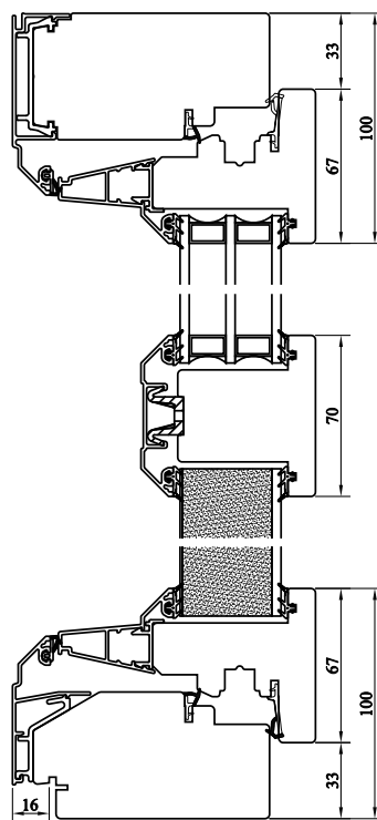
Vertikalsnitt
