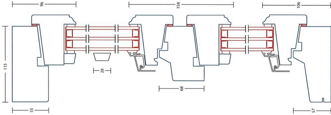
VERTIKALSNITT
