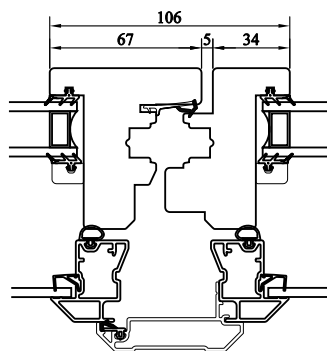
Horizontalsnitt pardörr
