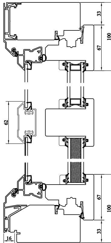
Vertikalsnitt
