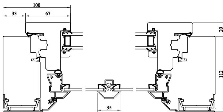
Horizontalsnitt
